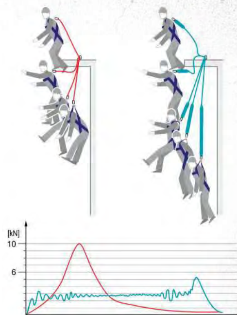
Slika 1. Poređenje apsorber energije i užde
